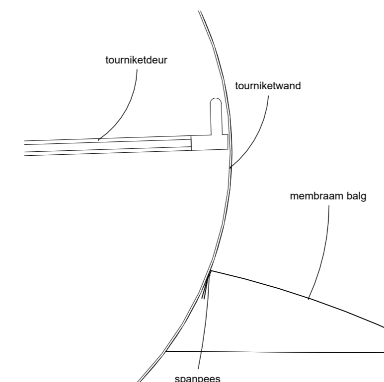
H2 Schaal: 1 : 10
