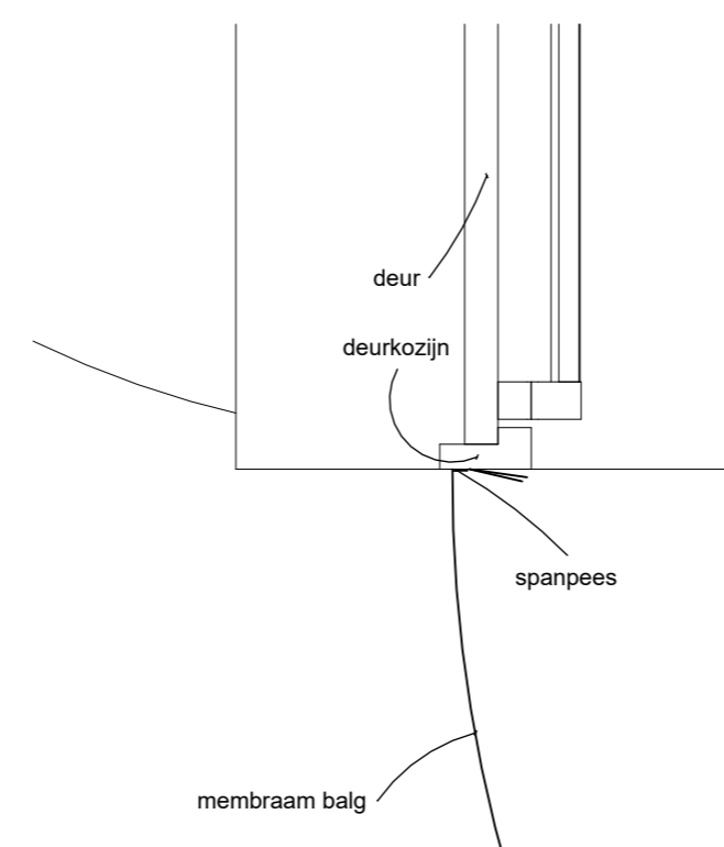
H1 Schaal: 1 : 10
